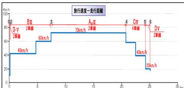
図-5 旅行速度－距離(目標とする階層)
