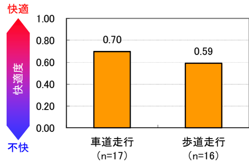
図4 車道及び歩道走行のLP面積による快適性評価
