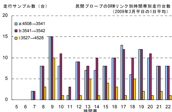
図-6 DRMリンク別時間帯別平均走行台数(平日平均)
