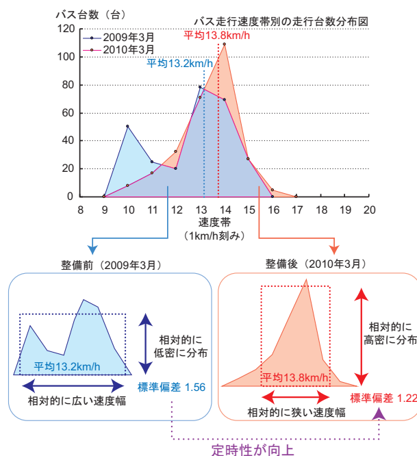
図-10 バス走行速度帯別の走行台数分布
