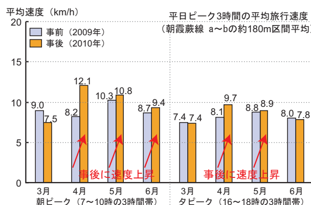
図-11 整備前後の時間帯別平均旅行速度の比較結果
