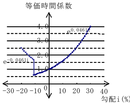
図1 勾配ごとの等価時間係数
