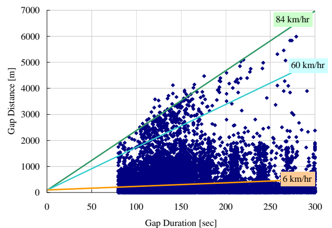
図1: 記録ギャップの継続時間と距離の関係(5分以下)
