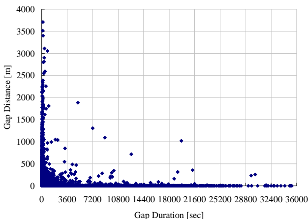
図 3：GPS 検出異常区間の継続時間と距離の関係
