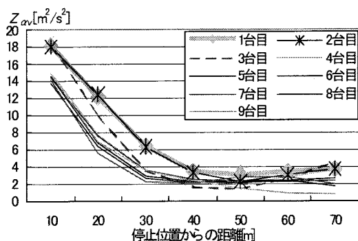
図-3 停止位置からの距離と Z_{av}
