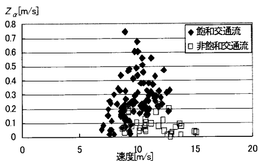
図-8 飽和と非飽和交通流時の Z_\alpha
