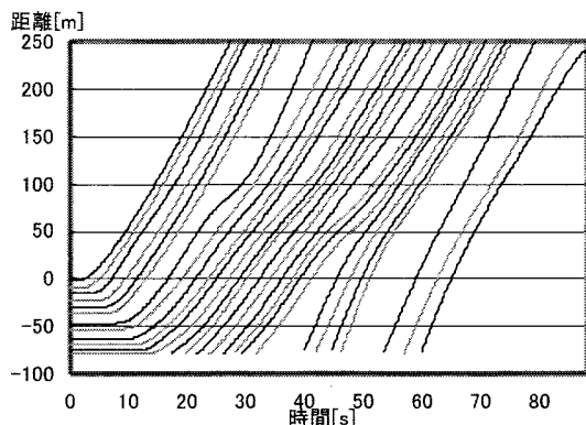
図-2 観測による車両軌跡
