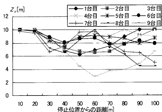
図-6 停止位置からの距離と Z_v
