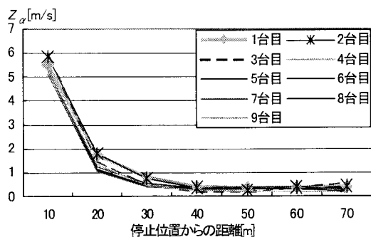
図-4 停止位置からの距離と Z_\alpha
