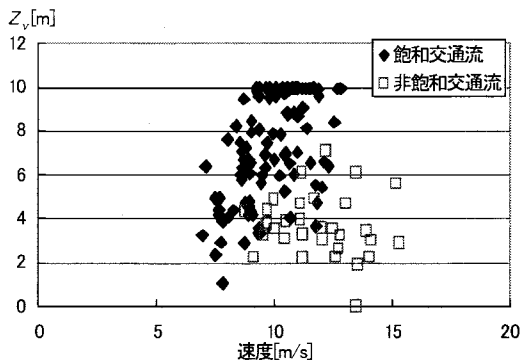
図-10 飽和と非飽和交通流時の Z_v
