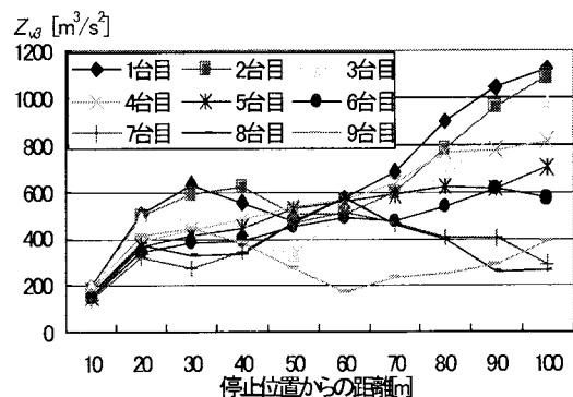
図-5 停止位置からの距離と Z_{v3}
