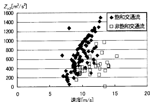
図-9 飽和と非飽和交通流時の Z_{v3}
