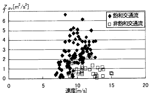
図-7 飽和と非飽和交通流時の Z_{av}
