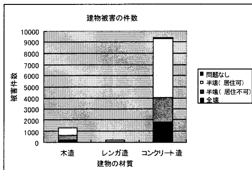
図-6. 建物の材質と倒壊度の割合
