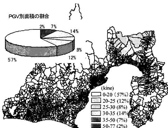
図-1 静岡県下の PGV 分布
