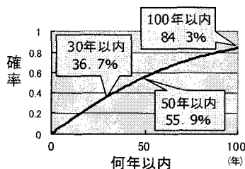
図－3 東海地震の発生確率
