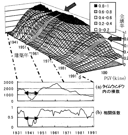
図 5 全壊率曲面
