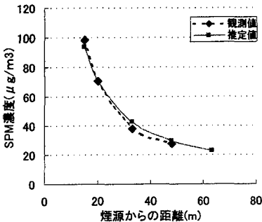
図7 線源パフモデルによる推定濃
