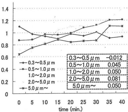
図2 降雨後の粒径分布
