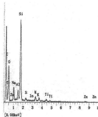
図10 SPM 成分元素
