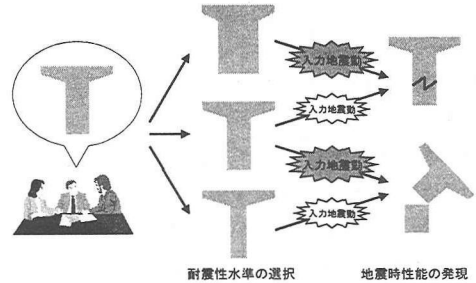
図1 耐震性水準、地震時性能の概念
