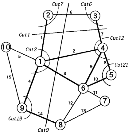
図-2 対象道路網と探索されたカット
