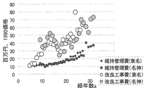
図4 純維持管理費の実績値の推移
