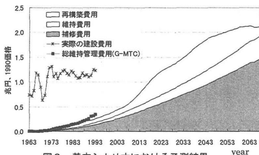
図6 基本シナリオにおける予測結果
