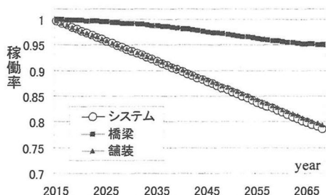
図9 財源不足シナリオによる稼働率の予測結果
