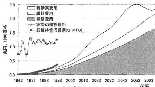
図7 建設集中シナリオ
