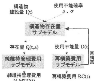
図2 モデルのフロー
