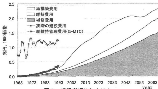
図8 橋梁老朽化シナリオ
