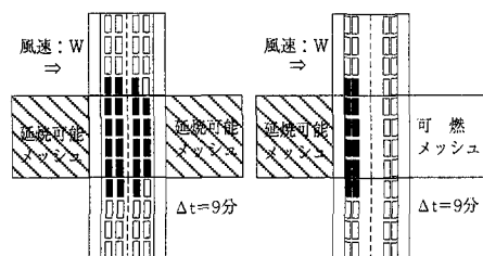
図6 車両火災算定事例 ( \Delta t=9\text{min} )
