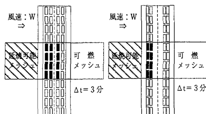
図5 車両火災算定事例 ( \Delta t=3\text{min} )
