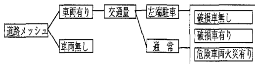
図1 道路メッシュの状態定義
