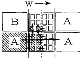
図2 道路メッシュ炎上パターン
