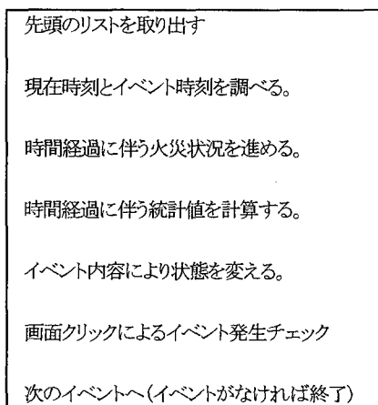
図3 イベント駆動のアルゴリズム
