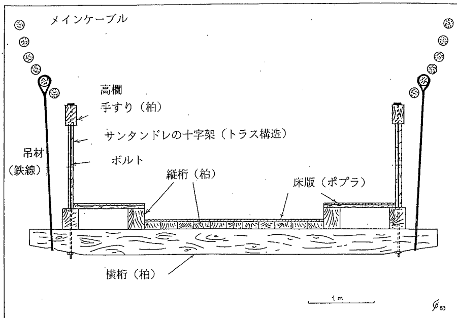
図-3 桁の断面図 (著者作成)
