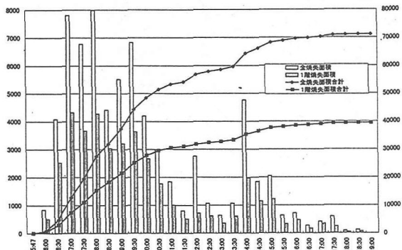
図5 若松町10丁目地区時刻別延焼面積
