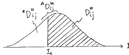
図3 立地需要に対する立地需要分布
