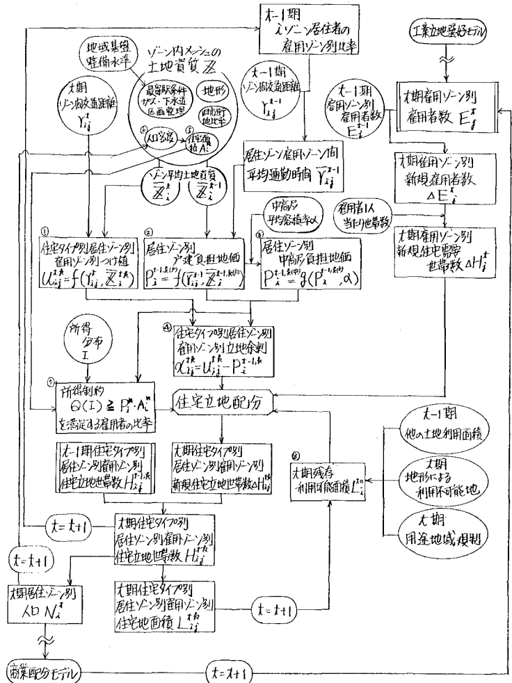
図2 住宅配分モデルフロー
