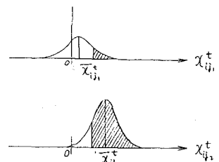
図5-c 時間と考慮した立地主体おおよびおの立地余剰の分布
