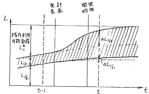
図5-b 立地主体おおよびおの立地量
