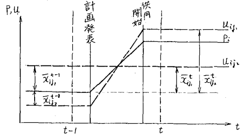
図5-a つけ値(u)、地価(P)、立地余剰の変化
