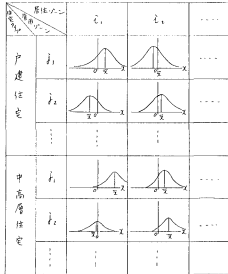
図3 立地需要に対する立地需要分布
