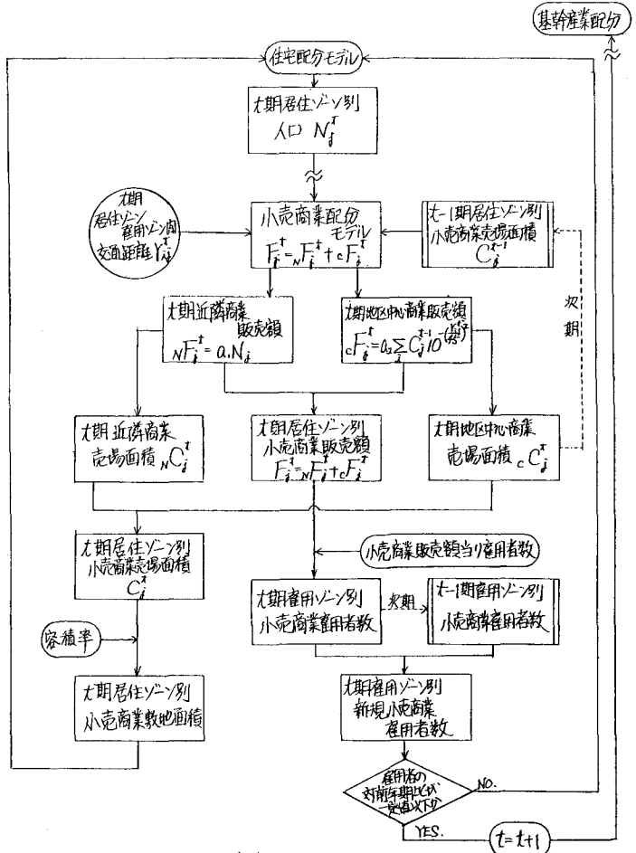
図6 小売商業配分モデルフロー
