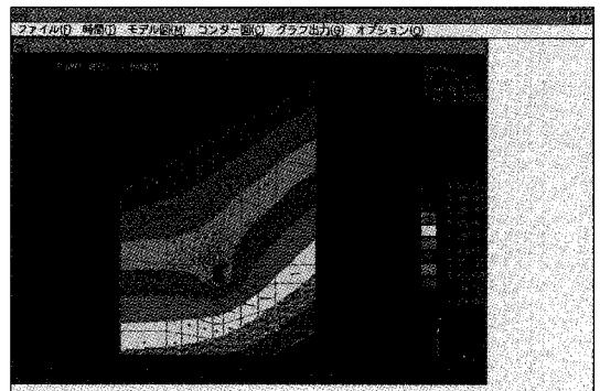
PC/UNISSF(V) : 圧力水頭コンター図と流速ベクトル図
