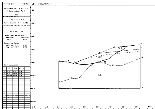
凸形基盤上の切土斜面
