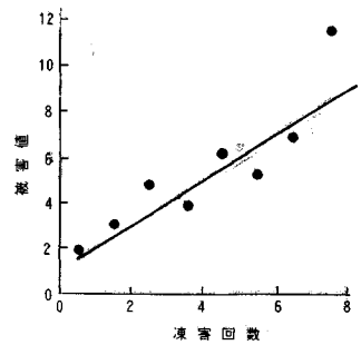
図-13 セメント協会方式(5)の検討(全橋梁) Max>0°C, Min≤-15°C
