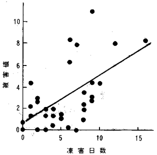
図-17 セメント協会方式 (2) の検討 (気象観測所) Max > 0°C, Min ≤ -10°C
