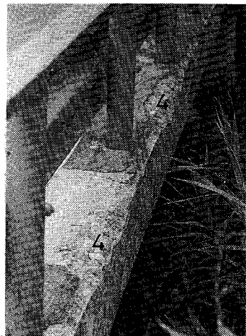
写真二 劣化の形態
