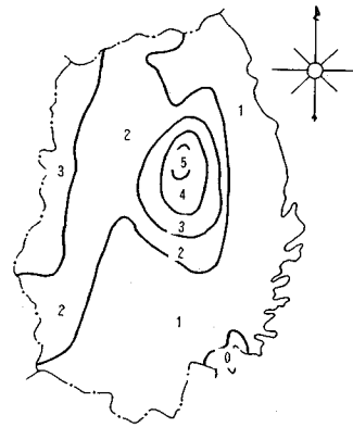
図一八 凍害危険度
