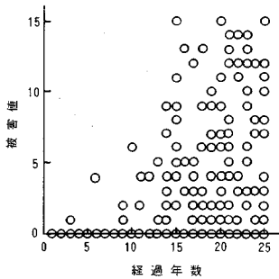
図-5 経過年数と被害値との関係
