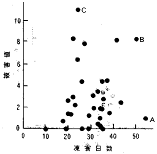
図-16 セメント協会方式 (1) の検討 (気象観測所) Max > 0°C, Min ≤ -5°C
