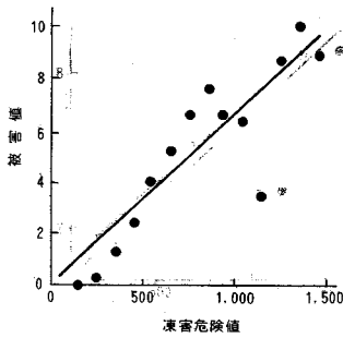
図-15 凍害危険値の検討 (全橋梁)
