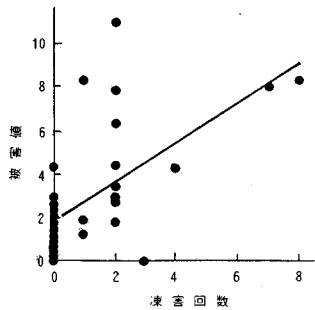
図-20 セメント協会方式 (5) の検討 (気象観測所) Max > 0°C, Min ≤ -15°C
