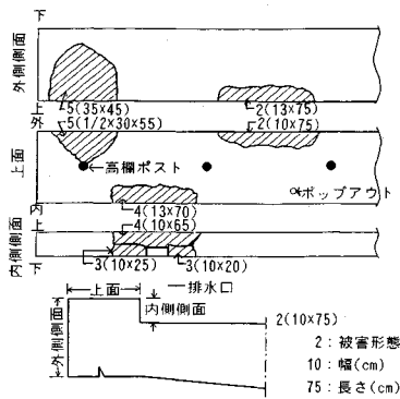
図一 地覆の劣化状況図
