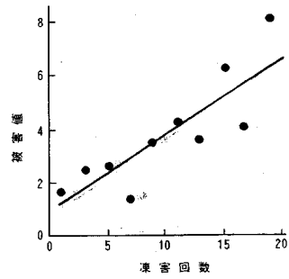
図-12 セメント協会方式(4)の検討(全橋梁) Max>0°C, Min≤-10°C
