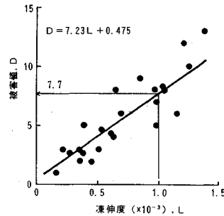
図-3 相対動弾性係数および凍伸度と被害値との関係
