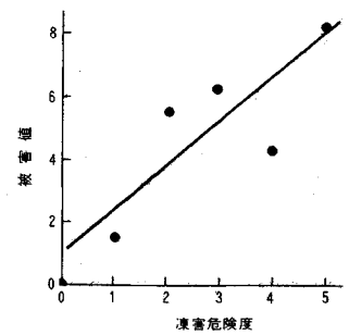
図-14 凍害危険度の検討(全橋梁)
