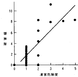
図—22 凍害危険度の検討（気象観測所）
