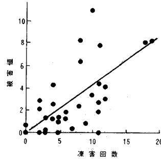
図-19 セメント協会方式 (4) の検討 (気象観測所) Max > 0°C, Min ≤ -10°C
