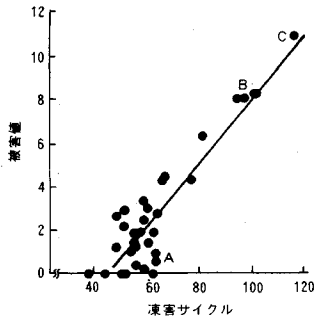
図-23 凍害サイクルの検討 (気象観測所)
