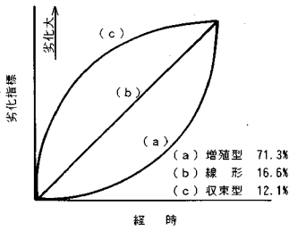
図-4 劣化の経時変化
