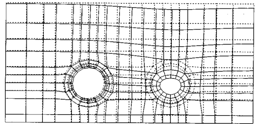
変形図
