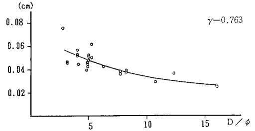
図一十九 鉄筋拔出し量と D/\phi の関係 (降伏時)
