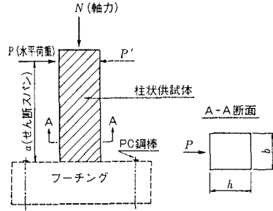
図-1 供試体形状
