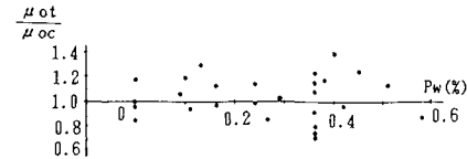
図-29 \mu_{ot} / \mu_{oc} と P 、 a/d 、 P_w との関係
