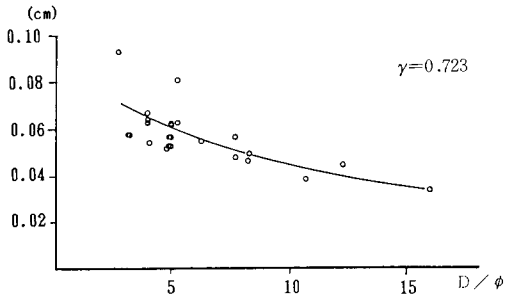
図一二十 鉄筋拔出し量と D/\phi の関係 (終局時)
