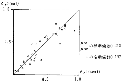
図-24 降伏時橋脚く体部分の変位 (cm)
