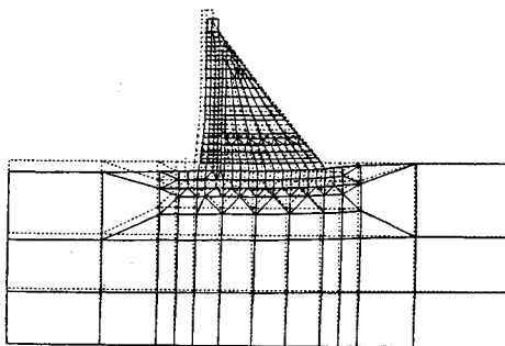
静水圧によるダム解析
