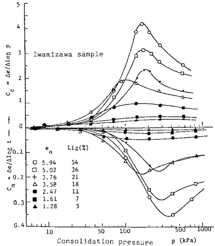
図一23 C_c と C_\alpha の圧密圧力依存性
