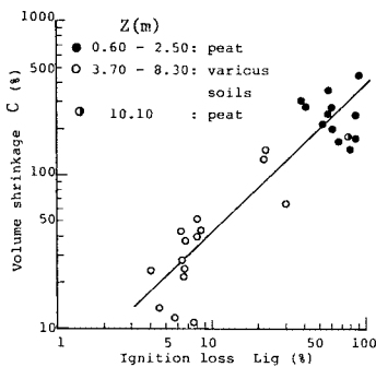
図-14 乾燥収縮による体積変化
