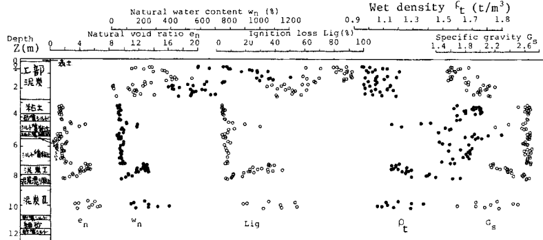
図-2 岩見沢泥炭地盤の土層構成と基本的性質の深さ方向の分布
