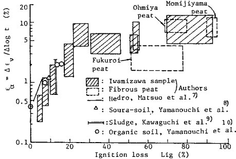
図—26 L_{1g} の相違による \epsilon_a の変化状況
