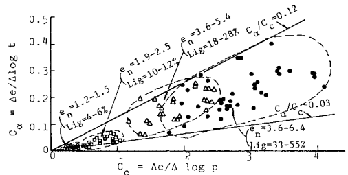
図一24 圧縮指数と二次圧密係数との関係
