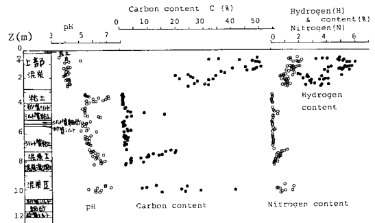
図-9 構成土層の元素分析結果
