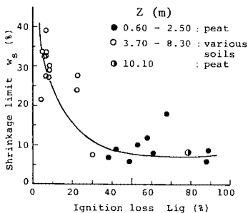
図-13 収縮限界と有機物含有量との関係
