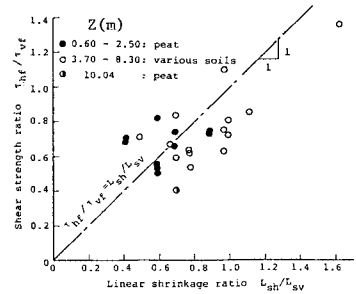
図一31 せん断強さと線収縮の方向性
