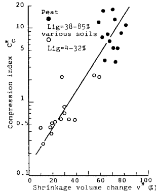
図一22 圧縮性と乾燥収縮性の関連
