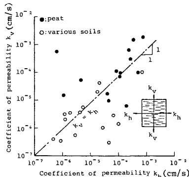
図—28 透水係数 ( k_v , k_h ) の方向性
