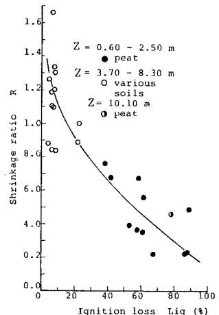
図-15 収縮比と有機物含有量との関係
