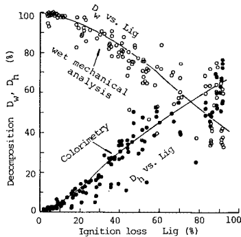
図-11 分解度 ( D_w , D_h ) と有機物含有量との関係
