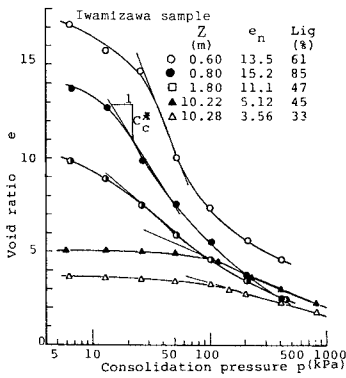
図一21 代表的試料の圧密曲線
