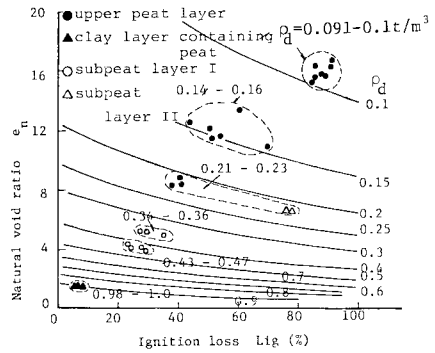
図-5 \rho_d をパラメーターとした e_n と L_{ig} との関係
