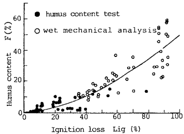
図-12 腐植含有量と有機物含有量との関係
