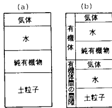
図-3 有機質土の相構成
