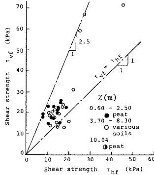
図一30 せん断強さの方向性
