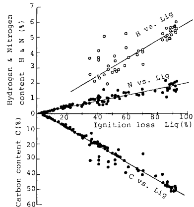
図-10 有機物含有量に占めるC, N, H含有量
