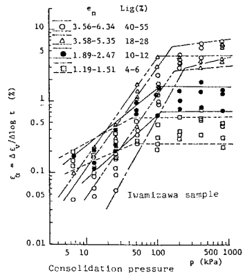
図一25 \epsilon_\alpha と圧密圧力との関係
