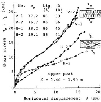
図一29 代表的泥炭試料の応力～変位曲線
