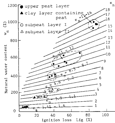
図-6 e_n をパラメーターとした w_n と L_{ig} との関係
