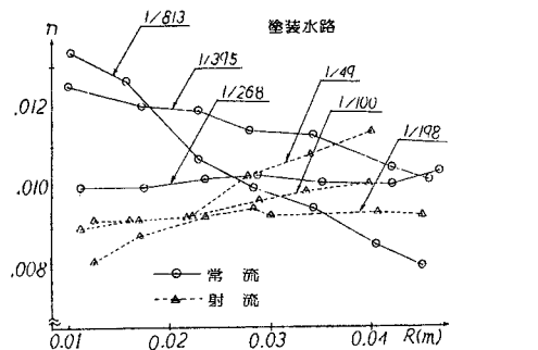
図一8 塗装水路での流雪能力実験結果(室内実験)
