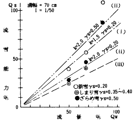
図-3 「流雪溝の運用と問題点」の実験結果 (一部)
