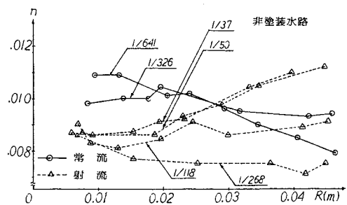
図一9 非塗装水路と塗装水路の粗度係数(18cm幅U字溝)
