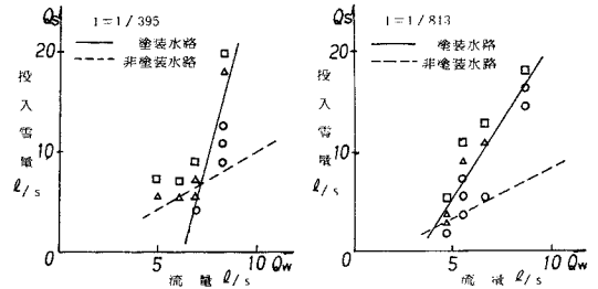
図一8 塗装水路での流雪能力実験結果(室内実験)
