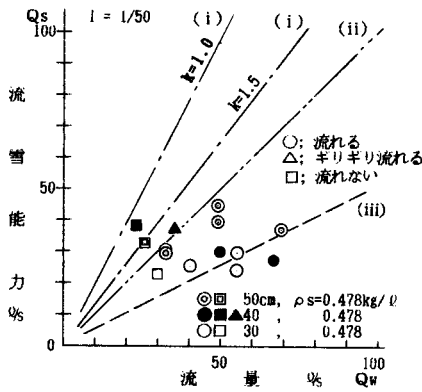
図-2 雪害実験研究所における実験結果 (一部)
