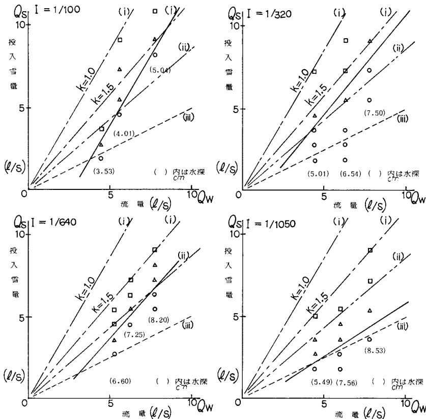
図一四 新潟大学における流雪能力に関する室内実験 (U字溝・幅18 cm)
