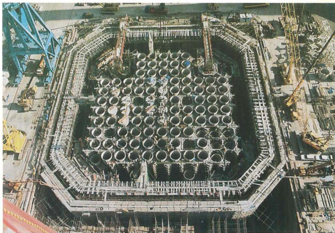
写真-2 浮体コンクリート建設時
