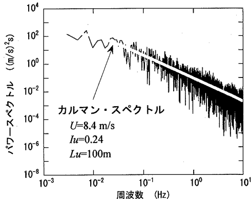
図-10 図-9 のパワースペクトル
