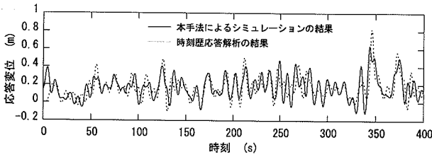
図-17 ピークファクターが小さく評価されてしまったシミュレーション結果の一例
