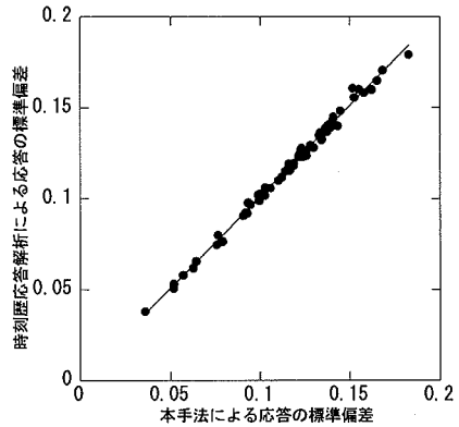
図-15 本手法と時刻歴応答解析とのガス応答変位の標準偏差に関する比較
