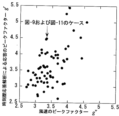
図-12 “風速のピークファクター” g^w と時刻歴応答解析により得られた応答のピークファクター g との比較
