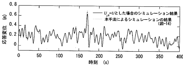
図-18 U_{j,k}=U とした場合のシミュレーション結果の一例
