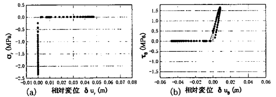
図-5 \theta = \pi/4 位置における境界点の履歴波形 (a) : r 方向、(b) : \theta 方向
