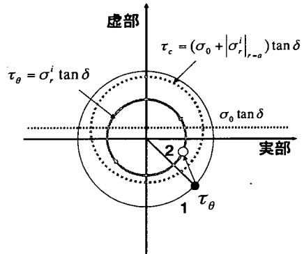
図-3 境界点で滑りが生じる場合のガウス平面上的特性
