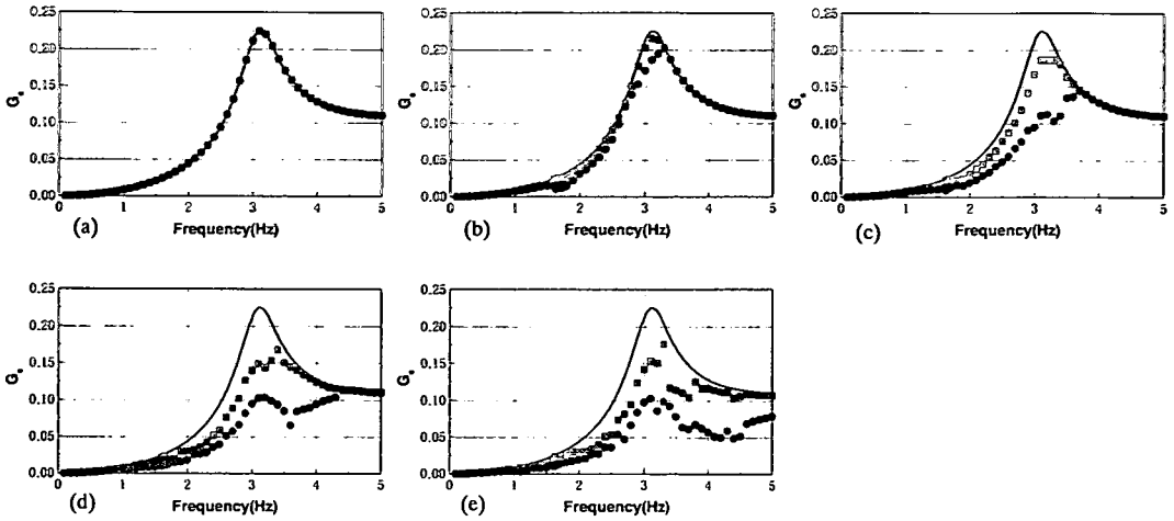
図-7 基盤入力加速度の変化に伴う無次元化作用土圧項の変化特性
