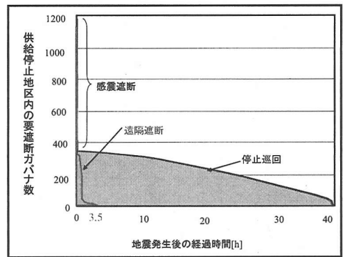
図-5 供給停止に要する時間の比較
