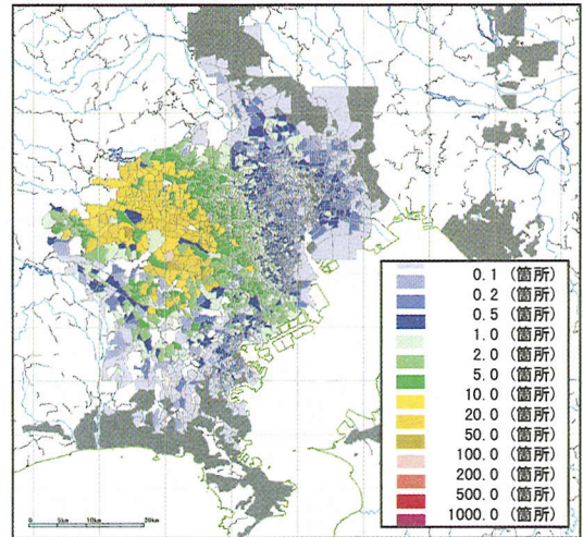
図-25 推定被害箇所数Mブロック集計(全管種) (想定立川断層地震)
