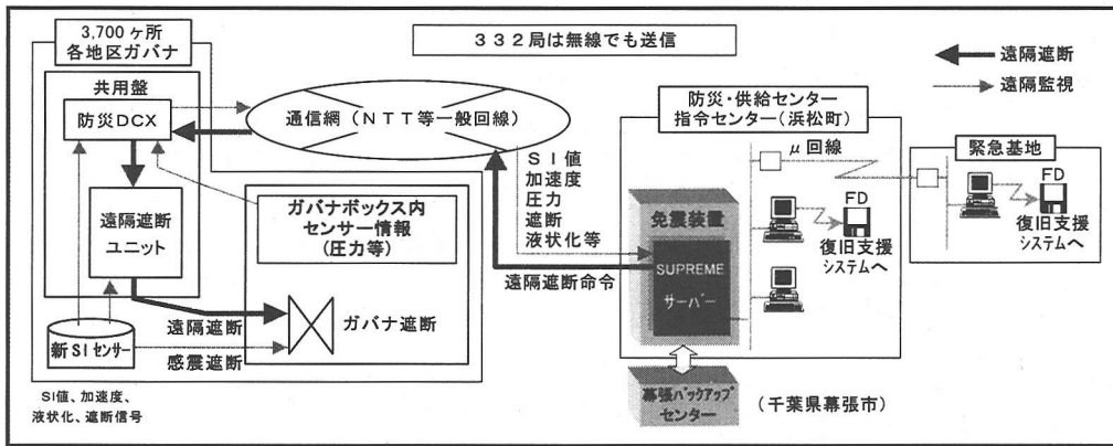
図-1 超高密度リアルタイム防災システム (SUPREME) の構成
