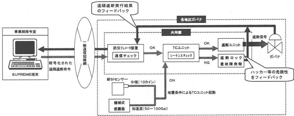
図-4 SUPREMEにおける地区ガバナ遠隔遮断安全性確保の仕組み
