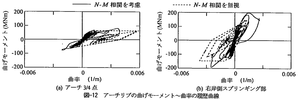
図-12 アーチリブの曲げモーメント～曲率の履歴曲線
