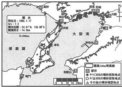
図-18 1995年兵庫県南部地震における噴砂採取地点 33)
