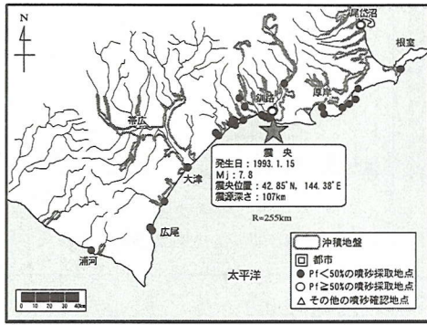
図-8 1993年釧路沖地震における噴砂採取地点 17)
