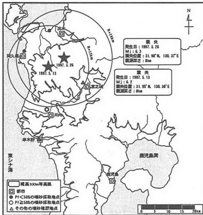
図-20 1997年鹿児島県北部地震における噴砂採取地点 34)
