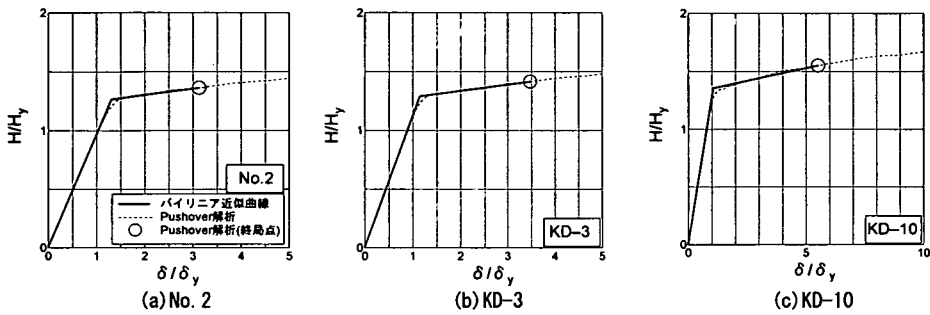
図-11 Pushover 解析結果，終局変位および推定復元力特性
