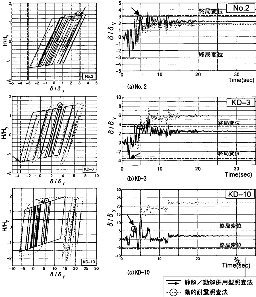
図-12 静的/動的解析併用照査法と動的照査法の推定結果の比較
