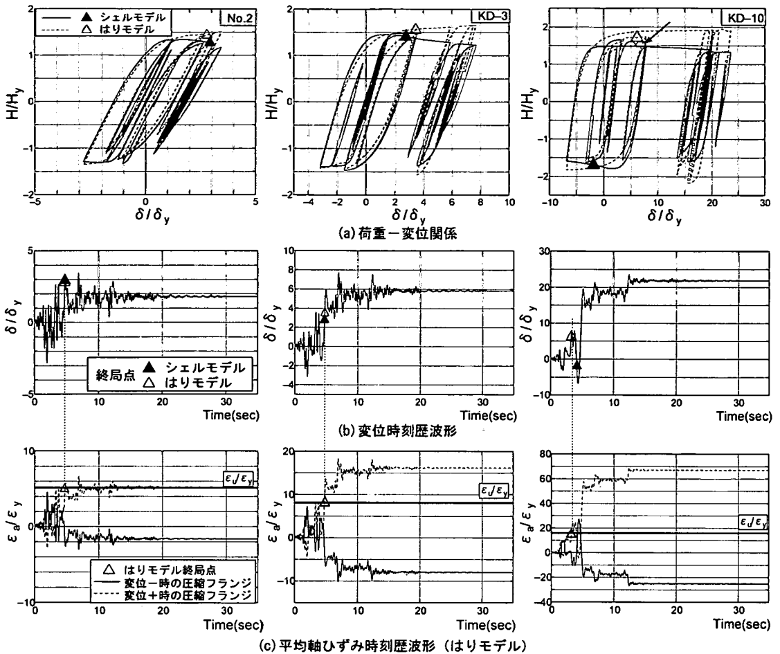
図-8 動的地震応答解析結果
