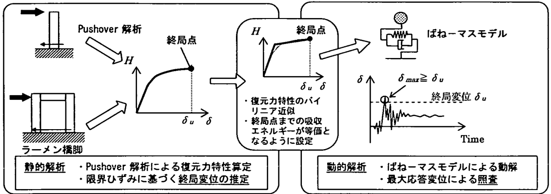
図-10 静的／動的解析併用型照査法概念図
