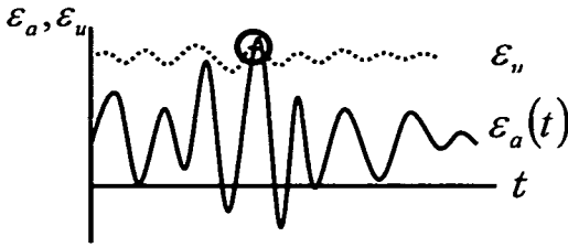
図-1 動的耐震照査法のご概念図
