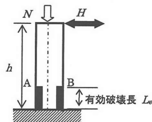
図-3 解析モデル概念図
