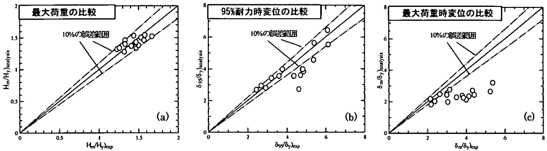
図-5 実験値と解析値の比較
