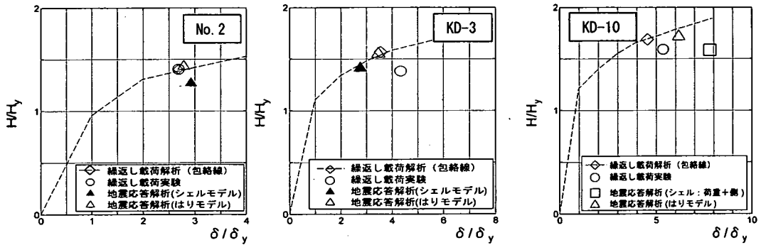
図-9 各評価における終局変位の比較
