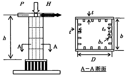
図-2 供試体概念図
