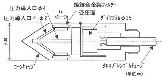
図-7 間隙水圧計の構造
