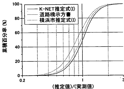
図-10 K-NET データに対して各推定式を使用した場合の S 波速度の(推定値)/(実測値)の累積分布
