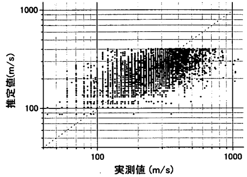
図-4 K-NETのS波速度実測値とK-NET推定式(I)によるS波速度推定値の関係
