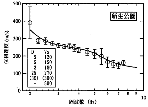
図-15 常時微動アレー観測から得られた観測位相速度と推定地盤構造
