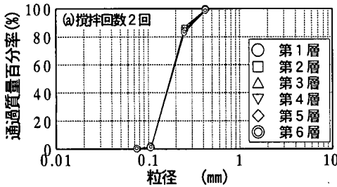
図-2 実験材料
