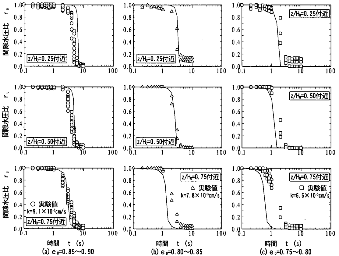
図-16 体積圧縮係数を変化させた逐次計算結果
