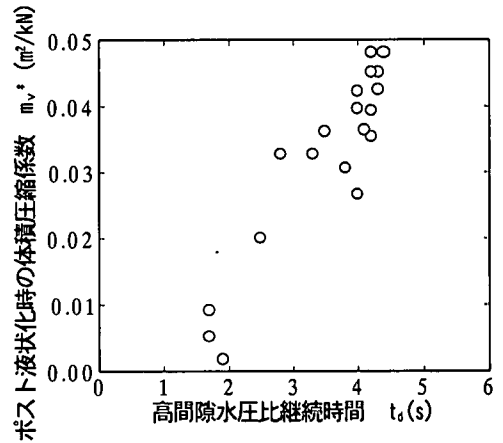
図-13 高間隙水圧比継続時間と液状化後の体積圧縮係数
