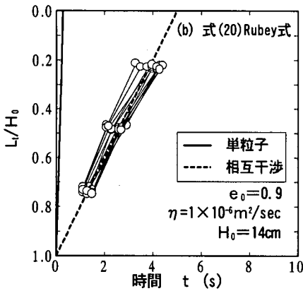
図-20 ポイリング領域の時間変化
