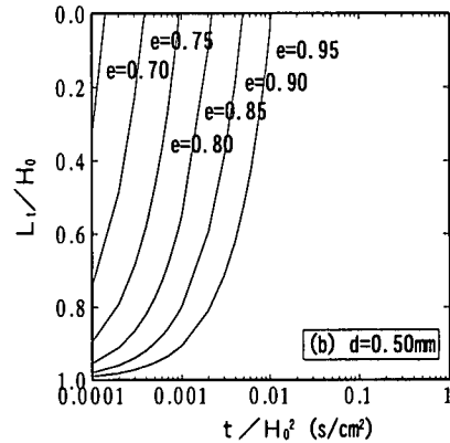
式(20)Rubey式 (相互干渉考慮)
