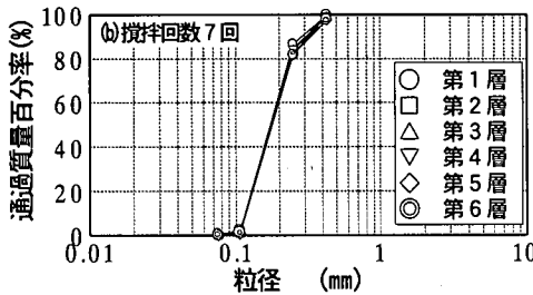
図-3 実験回数と分級の影響
