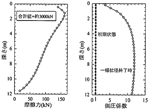
図-9 深さ～摩擦力分布
