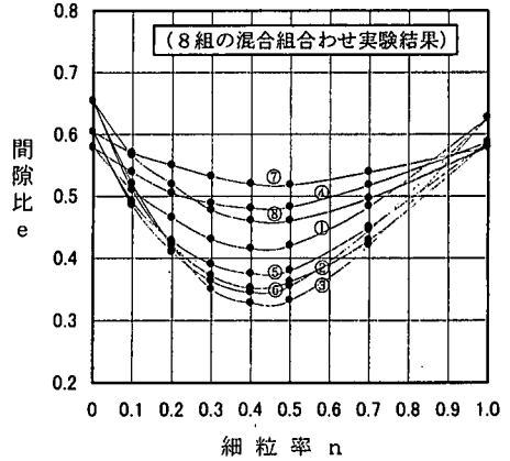
図-2 細粒率と間隙比の関係
