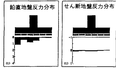
(a) 水平載荷力 H=511kgf
