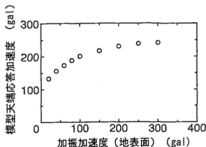
図-9 入力加速度と模型先端応答加速度の関係 (CASE2-60, 5.0Hz加振)
