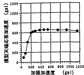
(c) CASE4-90-3 (土被り=1.0B)
