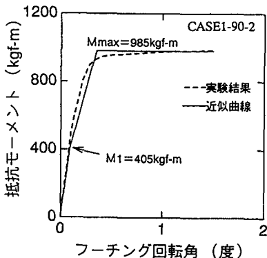
図-7 実験結果と近似曲線の比較 (CASE1-90-2)
