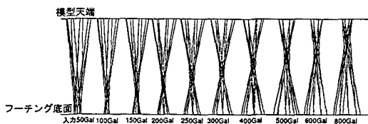
(b) CASE4-90-2 (土被り=0.5B)
