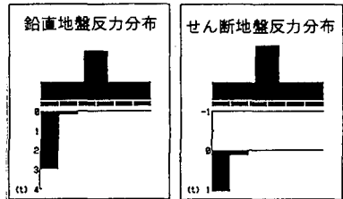
(d) 水平載荷力 H=1201kgf
