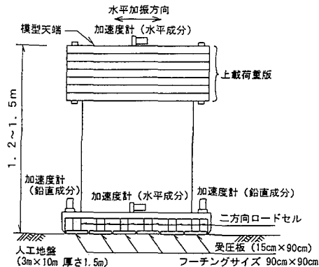
図-8 直接基礎模型概要
