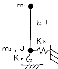
図-22 動的解析で考慮するモデル
