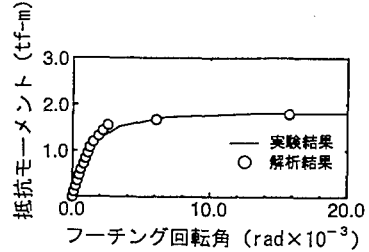
(a) CASE3-90-2の結果の比較
