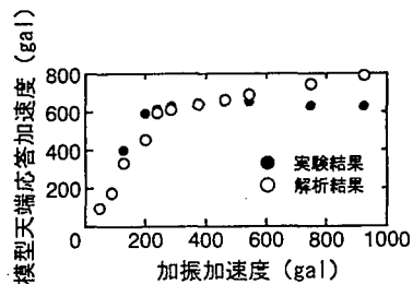
(c) CASE4-90-3の結果の比較
