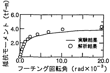
(b) CASE3-90-3の結果の比較
