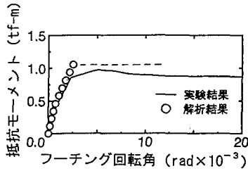
図-20 静的実験結果のシミュレーション(CASE3-90-1)
