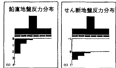
(c) 水平載荷力 H=1092kgf
