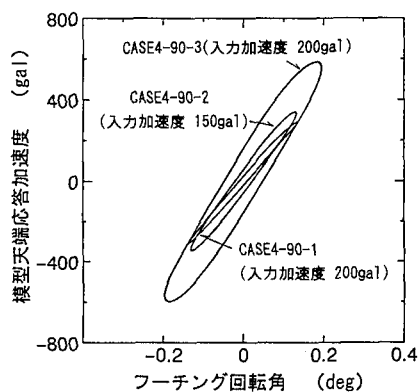
図-17 履歴ループ形状の比較
