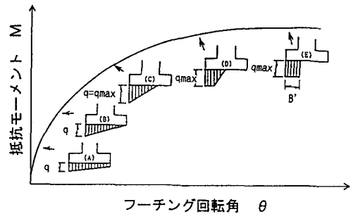
図-5 地盤反力形状の変化
