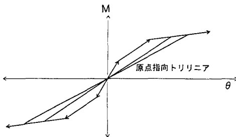
図-23 CASE4-90-1で考慮する回転ばねの履歴特性
