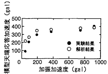
(a) CASE4-90-1の結果の比較
