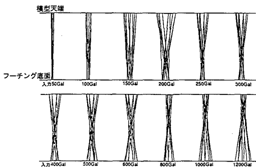
(c) CASE4-90-3 (土被り=1.0B)
