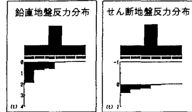
(b) 水平載荷力 H=953kgf
