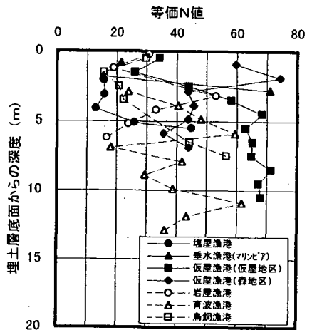
(b)基礎地盤の等価N値の深度分布図
