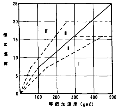
図-10 等価N値と等価加速度による液状化の判定図
