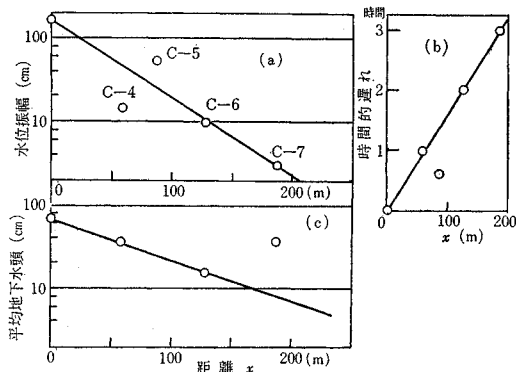
図-5 水位振幅、時間的遅れ、平均地下水頭
