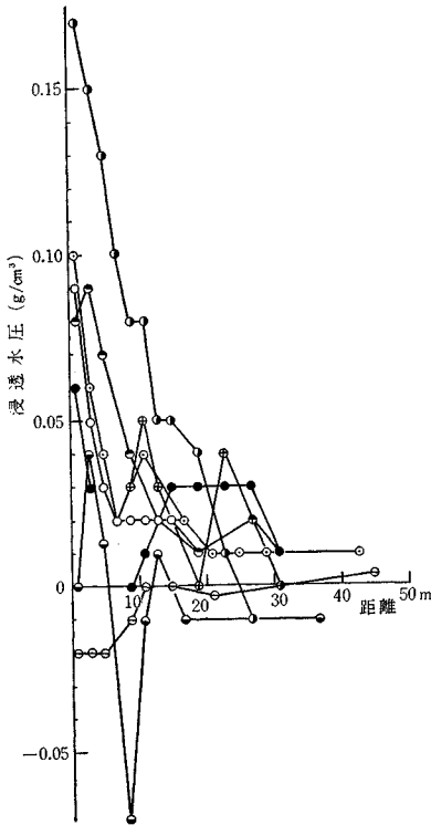
図-11 浸透水圧分布 (記号は図-10と同じ)
