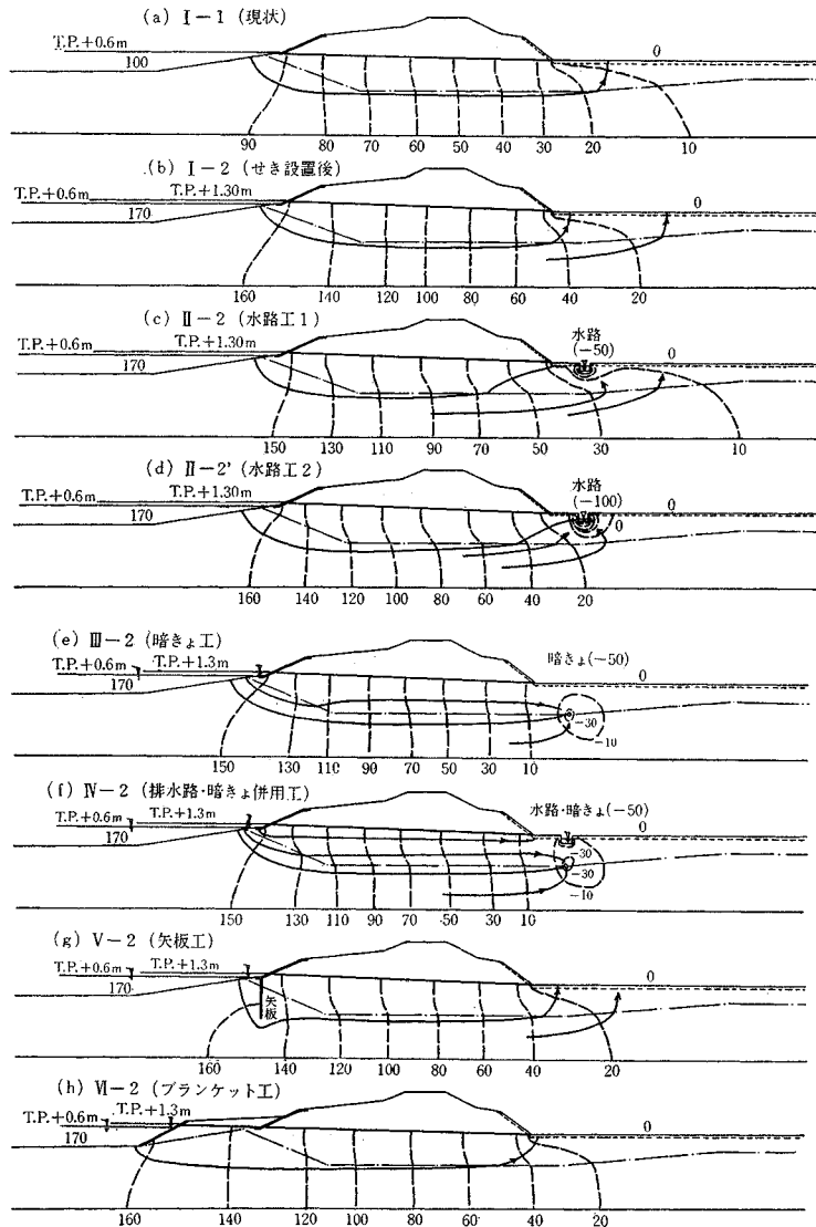
図-9 流線網
