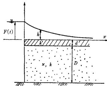
図-3 地盤モデル
