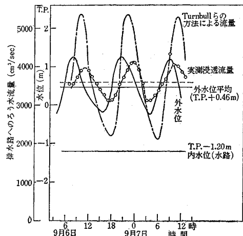
図-6 ろう水流量の変化
