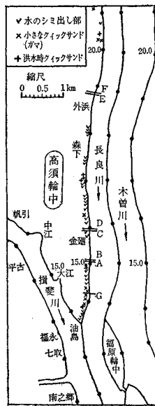
図-1 高須輪中平面図
