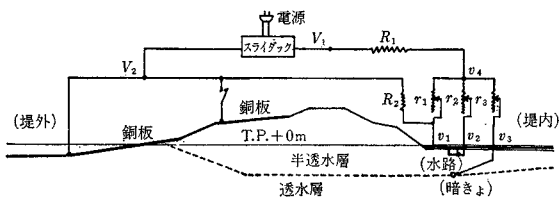
図-8 電気回路
