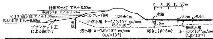
図-2 高須輪中堤防と地盤の断面(C断面)
