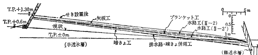
図-12 自由水面
