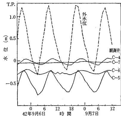
図-4 外水位と堤内地下水頭の変動
