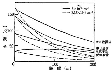
図-1 堤内地下水頭の分布(推定)
