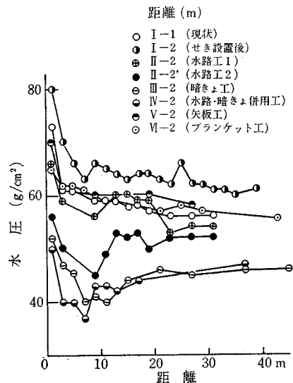
図—10 水圧分布
