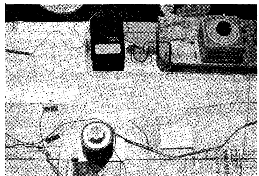
写真-1 寒天模型実験装置
