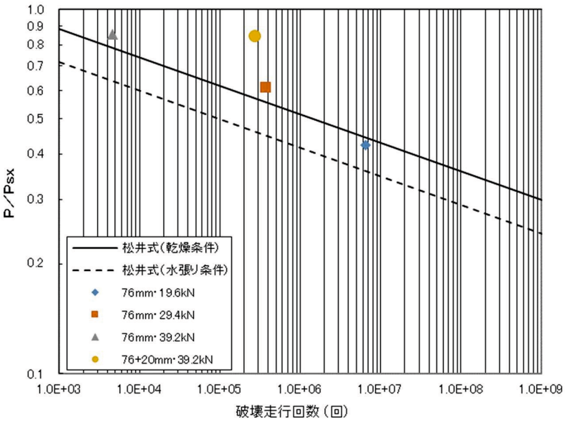
図 1 破壊走行回数と荷重比(P/P sx )の関係
