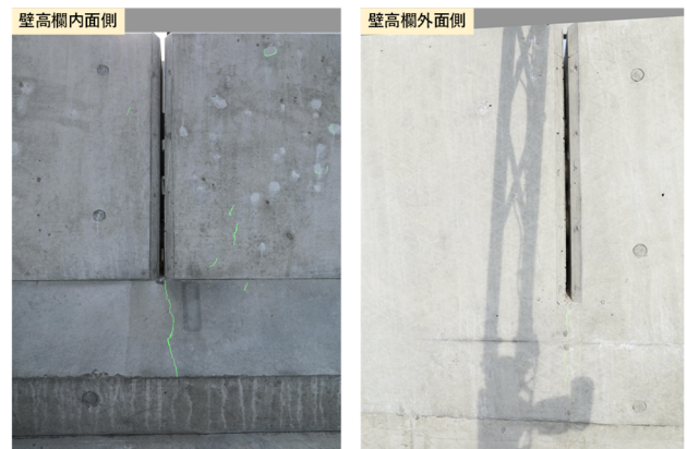
(b) 壁高欄
