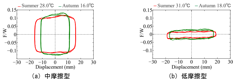
図-3 履歴曲線
