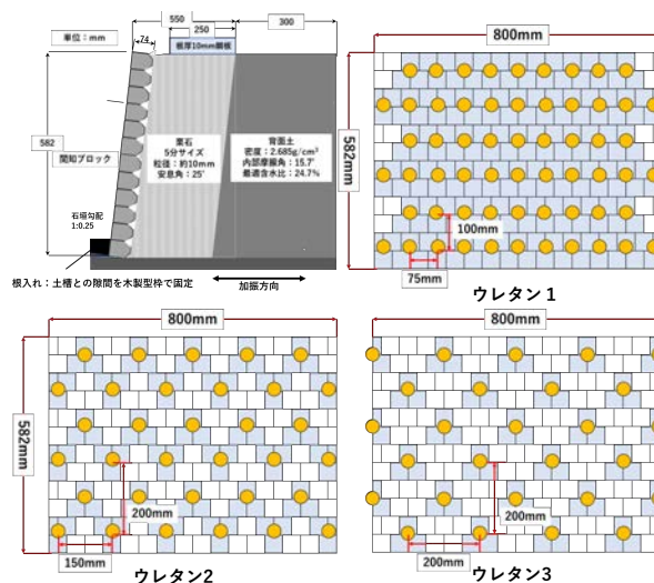
図1 側面における石垣モデルの概要と 各モデルのウレタン充填箇所
