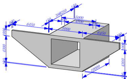
図-5 ウィングのモデル化および寸法表示例
