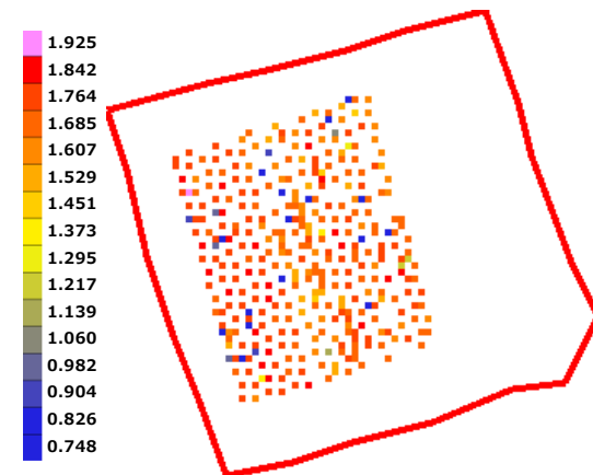
図-3 乾燥密度のヒートマップ
