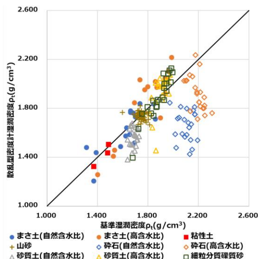
図-2 自動走行式散乱型 RI 密度計と透過型 RI の湿潤密度の相関
