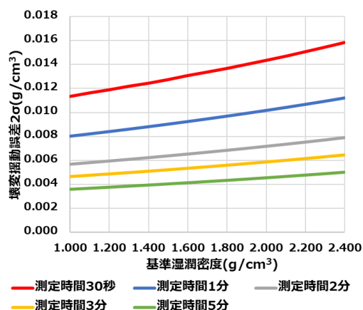
図-1 自動走行式散乱型 RI 密度計の壊変揺動誤差
