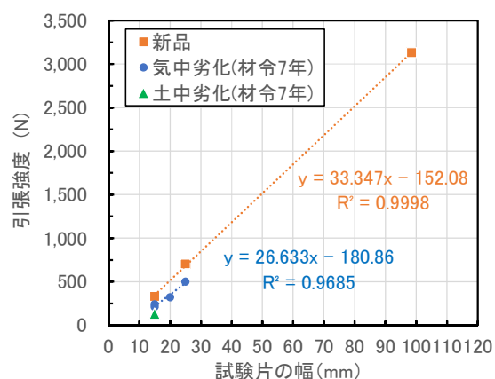
図-2 試験片幅とピーク強度の関係
