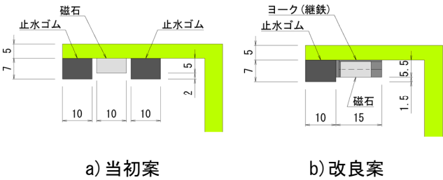
図-5 磁石による排水桝への固定方法
