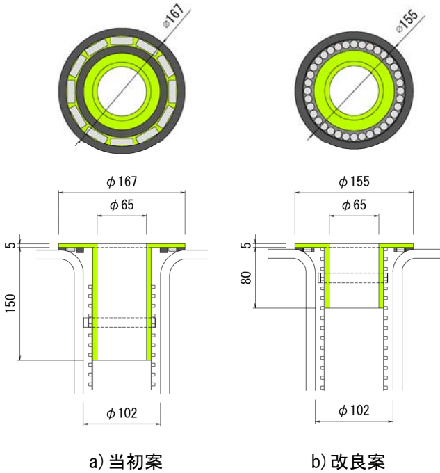
図-4 排水桝接合部の構造
