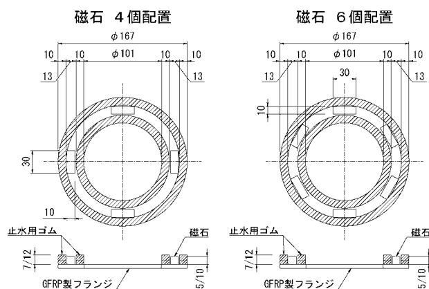
図-2 止水試験用 供試体
