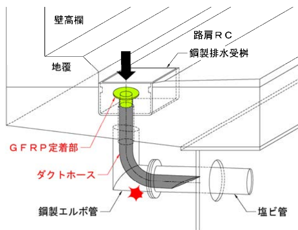
図-1 インサートノズル工法の概要
