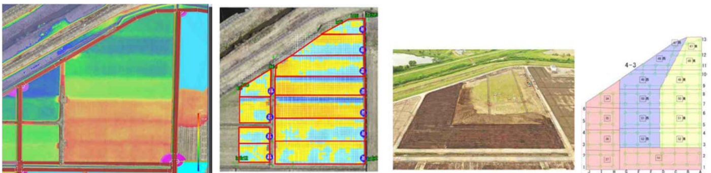
図 1：左から現況ほ場標高分布、セグメント毎平均標高算出、小規模施工エリア
